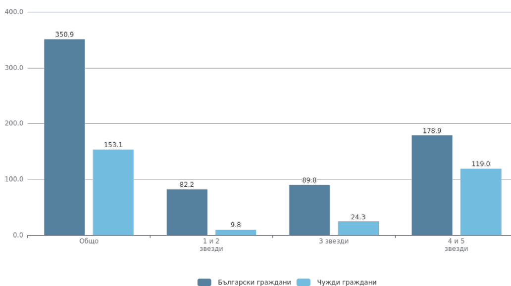
Фиг. 2. Пренощували лица по категории на местата за настаняване през февруари 2026 година
